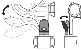
クイックカムロックシステム
