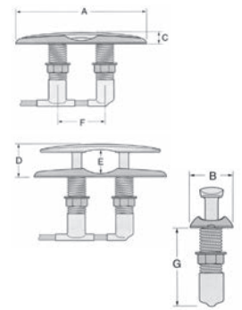
●ブルアップクリート (アップダウンクリート) SUS316
